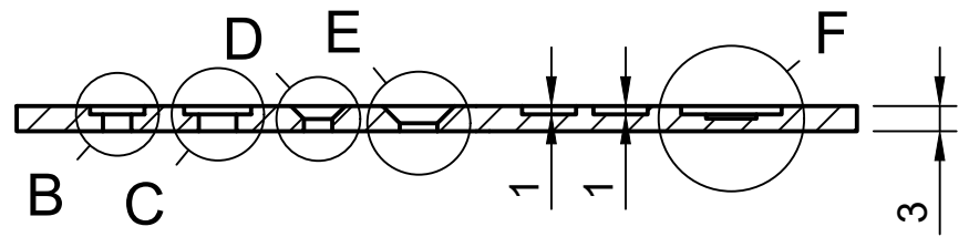
A-A (1:1)
